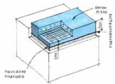
плитный
