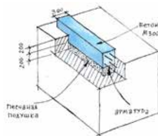
ленточный незаглубленный
